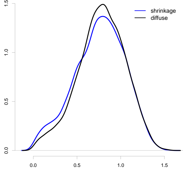
Figure 1: Marginal posterior densities of parameter B_{21}
